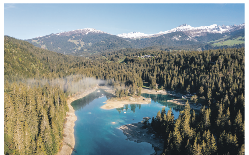
Caumasee
